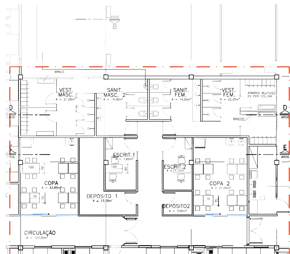
Planta baixa da Área de Apoio no pavimento térreo do Prédio da Administração Central
