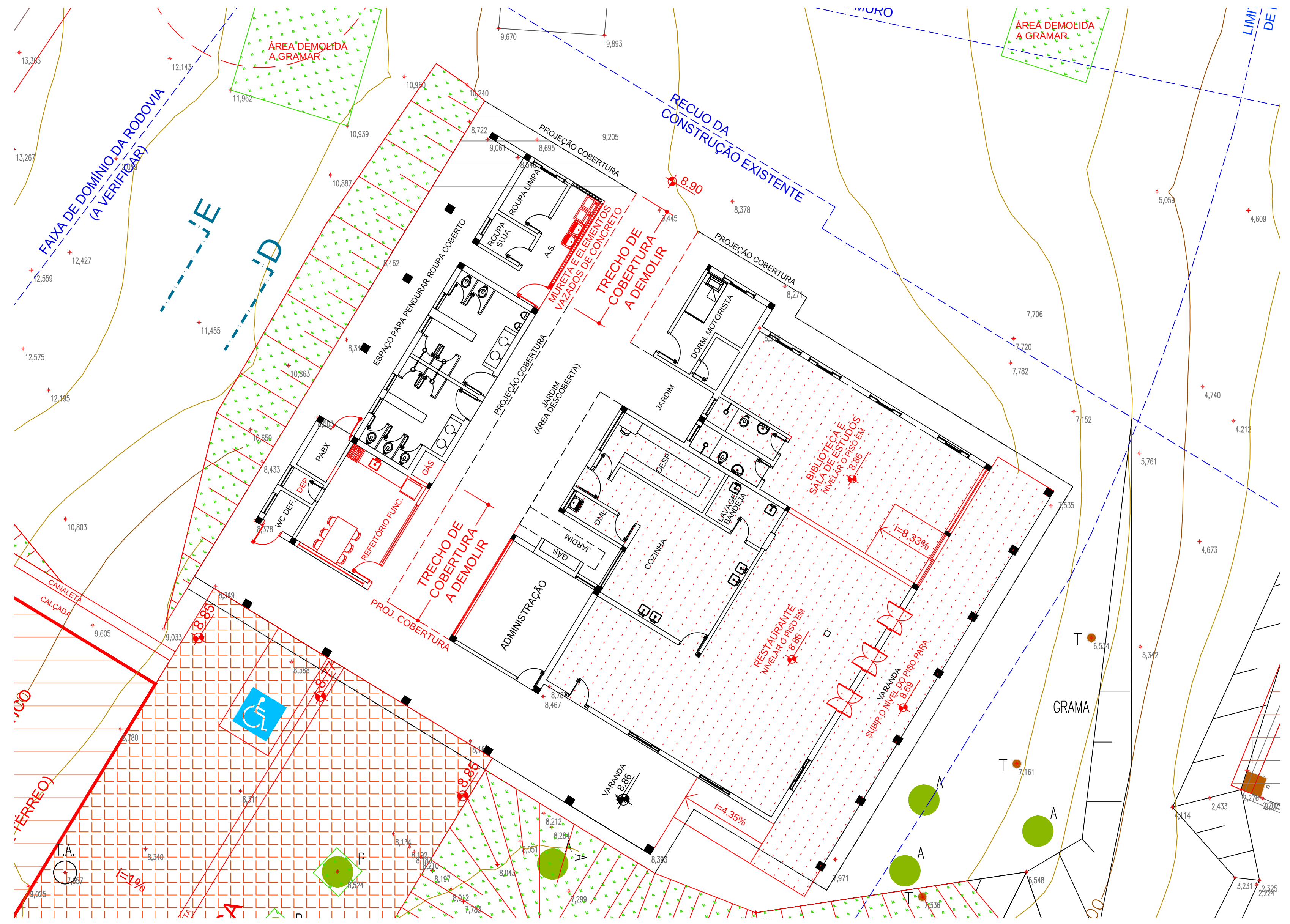
PROPOSTA 1ª ETAPA ESCALA: 1/125
