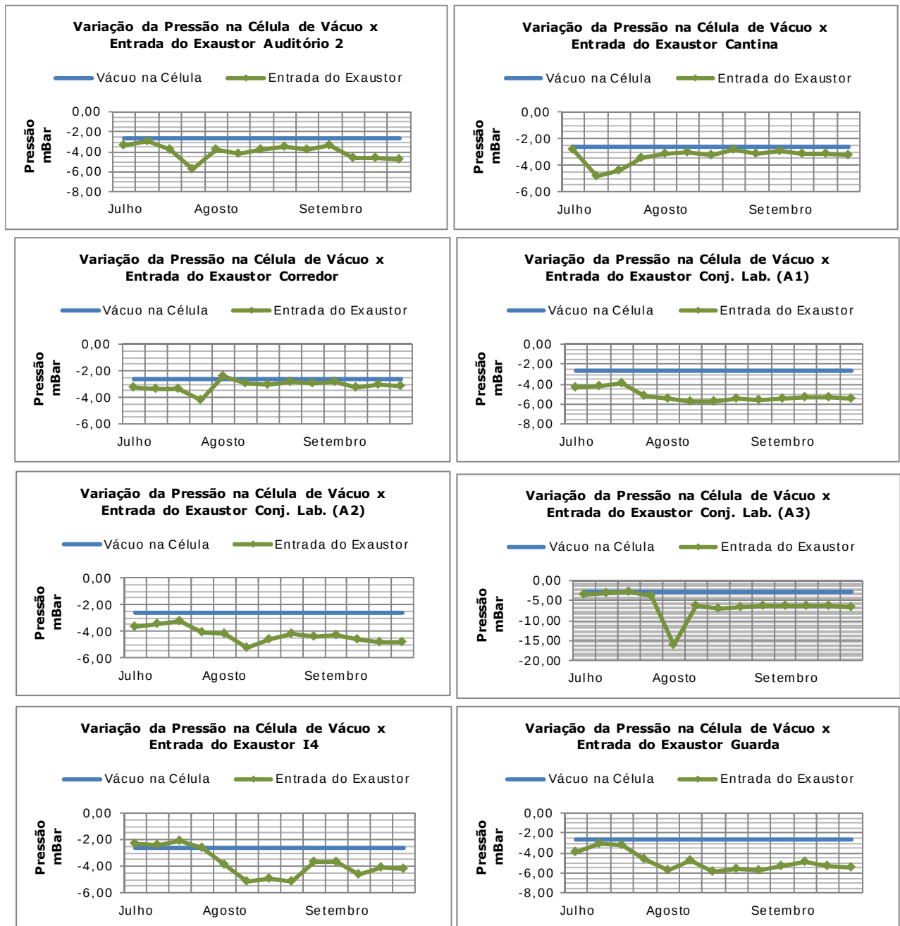
Gráficos de Variação da Pressão Célula de Vácuo x Entrada dos Exaustores Auditório 2, Cantina, Corredor, Conj. Lab. (A1), Conj. Lab. (A2), Conj. Lab. (A3), I4, Guarda
