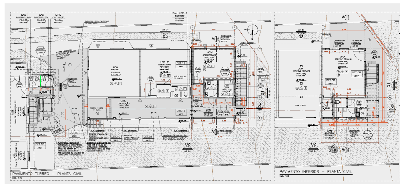
Planta baixa do térreo e planta baixa do pavimento inferior, com indicação da ampliação e demais intervenções
