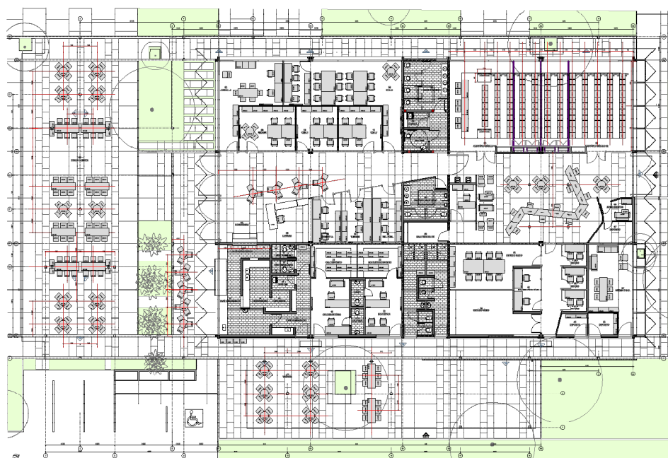
Planta baixa da reforma e das novas áreas externas cobertas
