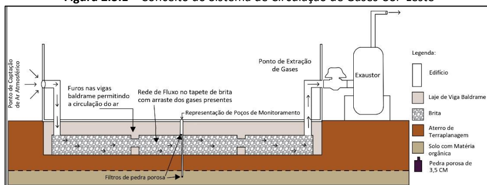
Figura 2.3.1 – Conceito do Sistema de Circulação de Gases USP Leste
