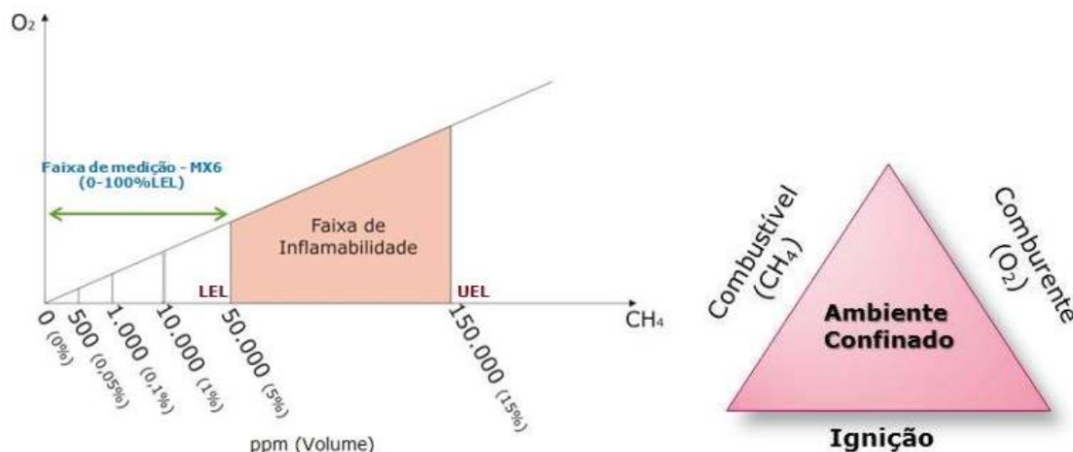
Figura 4.1.1. – Faixa de Inflamabilidade do Gás Metano ( CH_4 ) e sua Combustão
